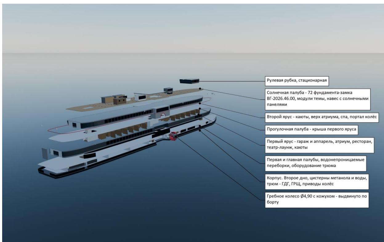
Рисунок 17 - Компонировочная схема (взрыв-модель)
