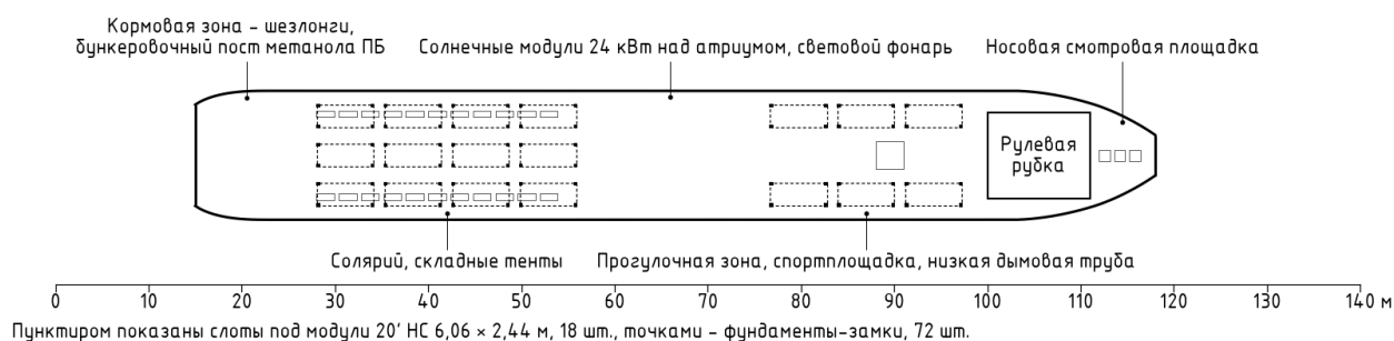
Рисунок 23 - План солнечной палубы
