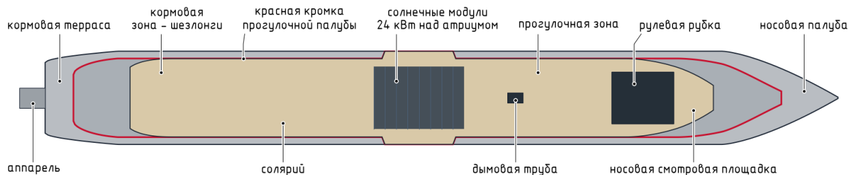
Рисунок 7 - Облик судна, вид сверху
