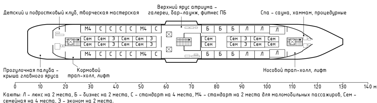
Рисунок 22 - План средней палубы
