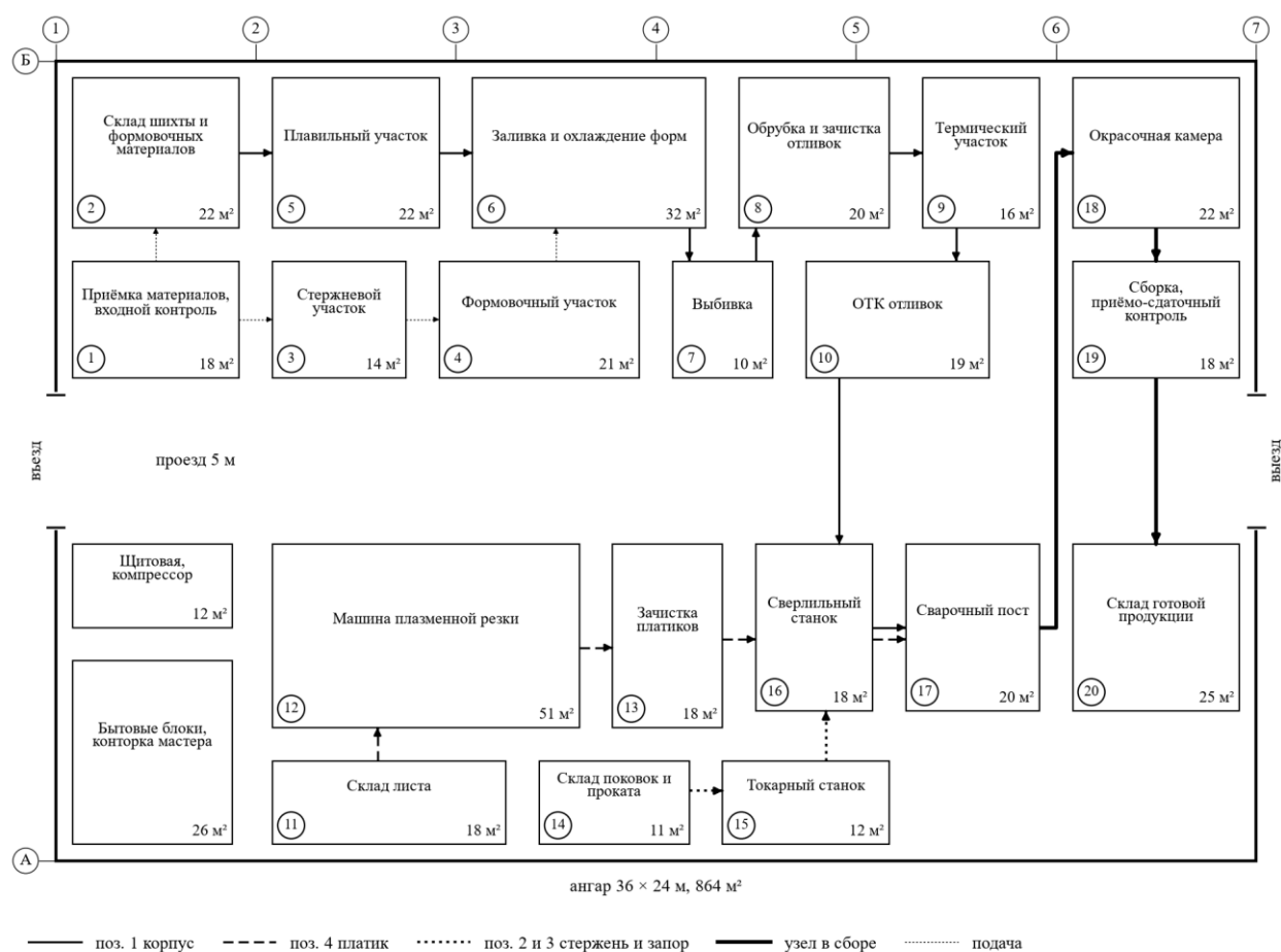
Рисунок 33 - Планировка цеха фундаментов в ангаре
