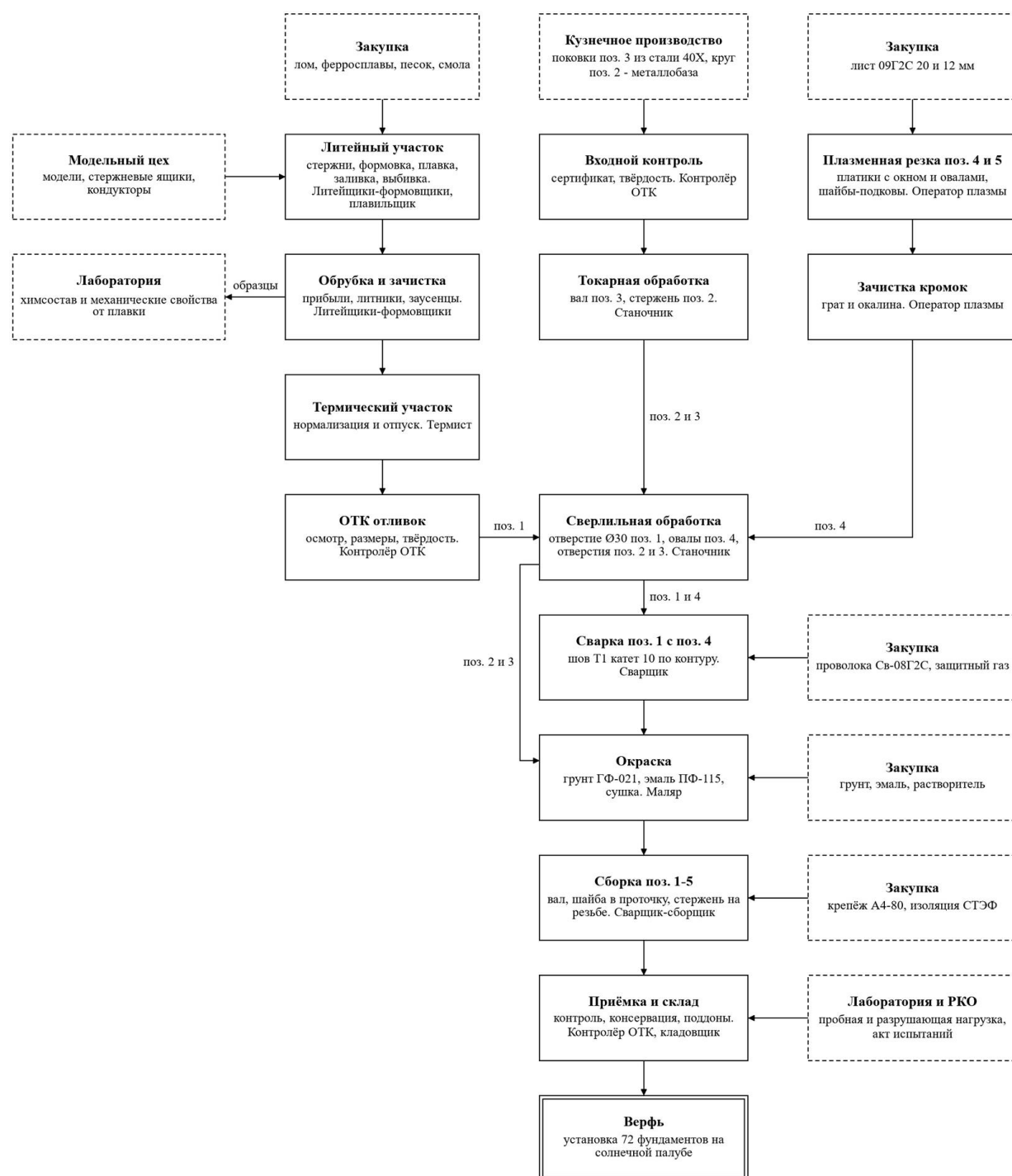
Рисунок 32 - Схема производства и кооперации узла
