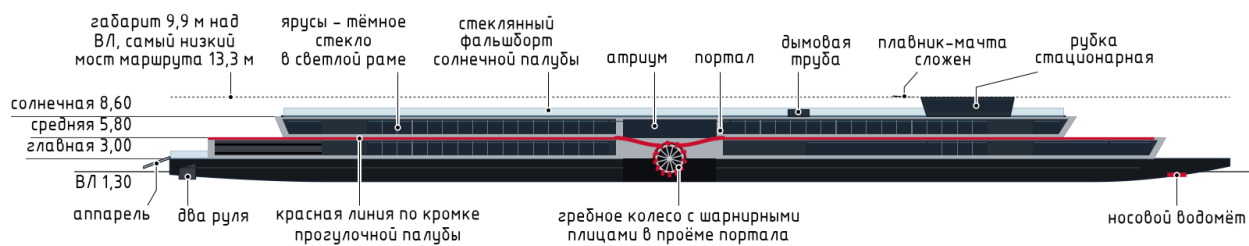
Рисунок 6 - Облик судна, вид сбоку
