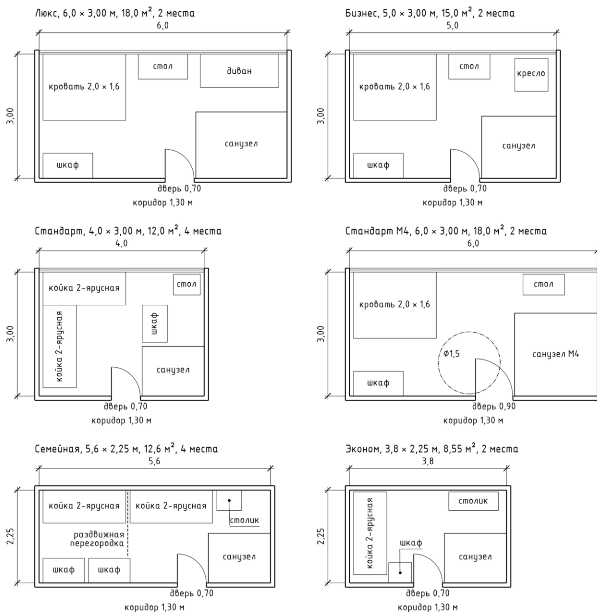
Рисунок 24 - Планировки кают шести типов
