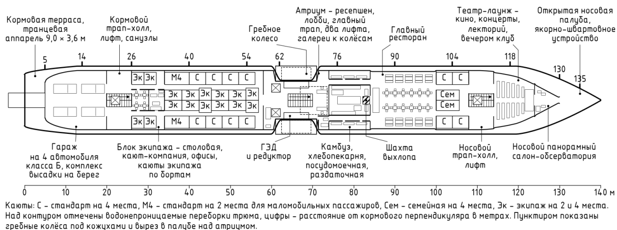
Рисунок 21 - План главной палубы
