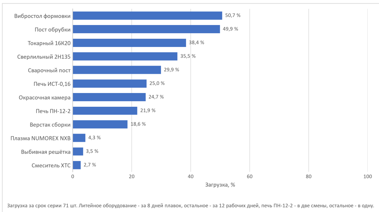
Рисунок 31 - Загрузка оборудования цеха серий фундаментов
