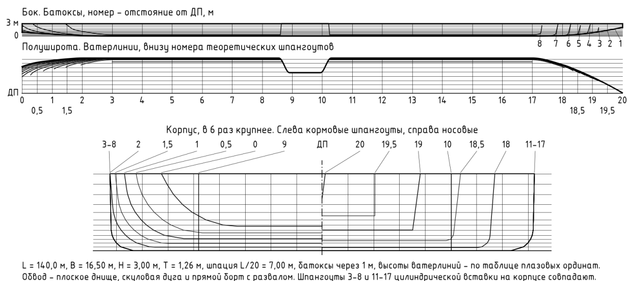
Рисунок А.1 - Теоретический чертёж
