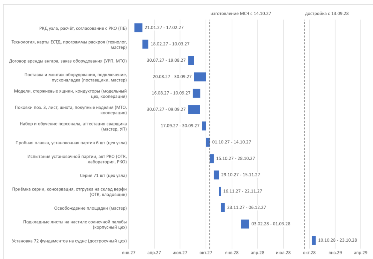
Рисунок 34 - Сроки подготовки и освоения производства фундаментов
